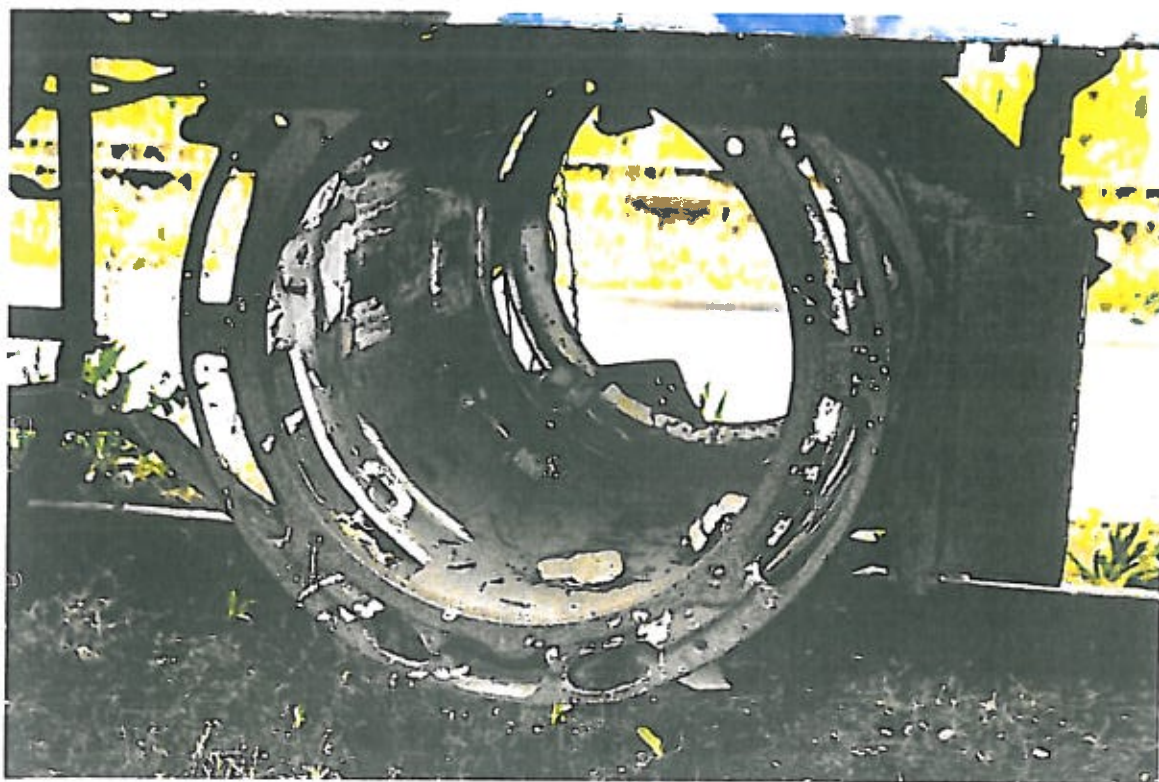
Rysunek 34: Pozostałości silnika umieszczone pod podłogą wagonu. Fot. P. Ratajczyk
