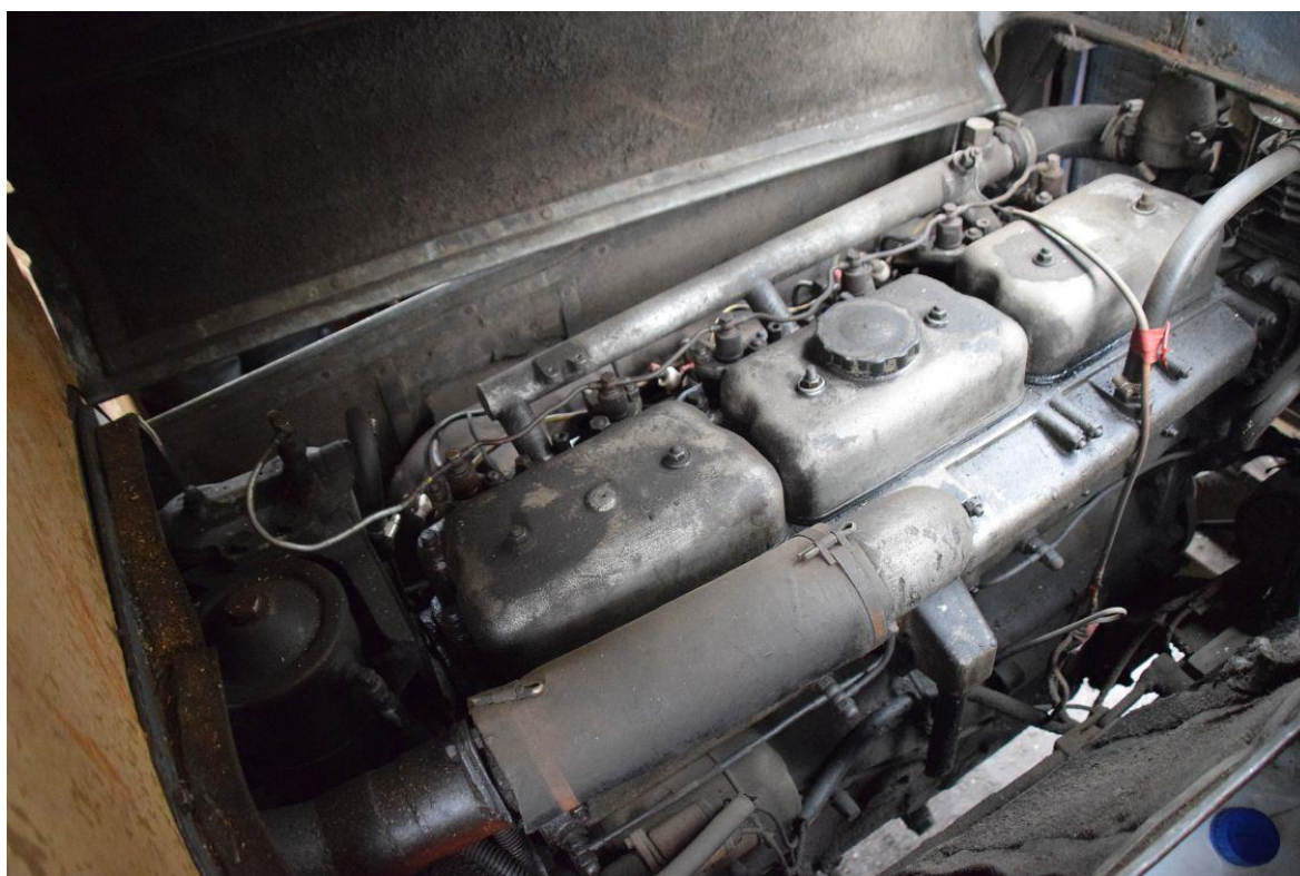
Fot. 12: Silnik wagonu spalinowego Mbd1-126 (W3M) nr inw. MUZ II 233, fot. Marta Przygoda-Stelmach
